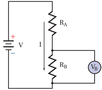
الشكل 4-8 في دائرة مجزئ الجهد
