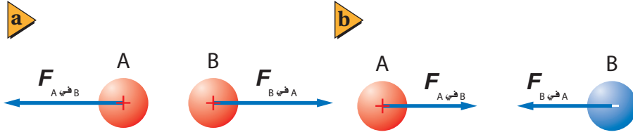
■ الشكل 13-5 قاعدة تحديد اتجاه القوة هي: الشحنات المتشابهة تتنافر؛ والشحنات المختلفة تتجاذب.
