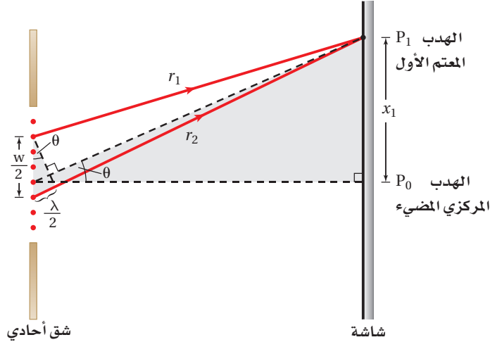
■ الشكل 10-4 يمثل هذا الرسم تحليلاً للهدب المعتم الأول. ويكون بعد الشق عن الشاشة L أكبر كثيراً من عرضه w .
