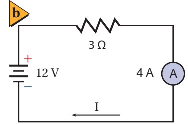
الشكل 7-7 يبين هذان الرسمان التخطيطيان دائرة توازي (a) ودائرة توالي (b) كهربائيتين.
