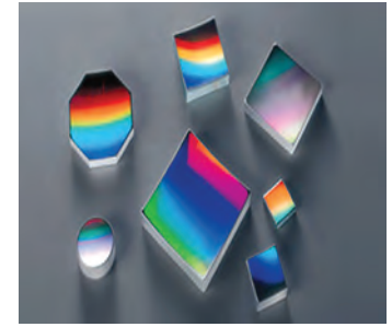
■ الشكل 11-4 تستخدم محزوزات الحيود لتكوين أنماط الحيود من أجل تحليل مصادر الضوء.
