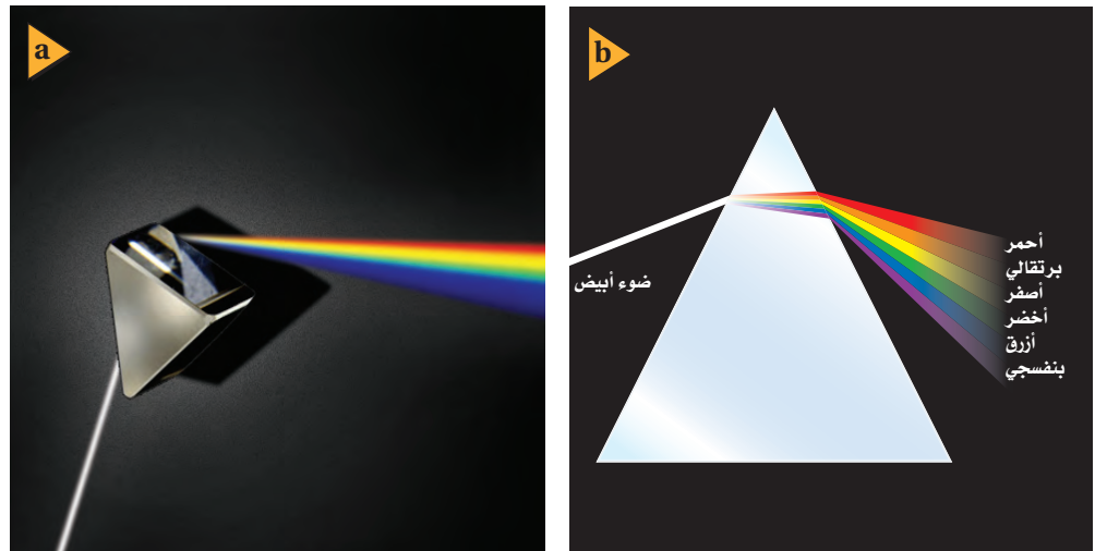
الشكل 3-6 يسقط ضوء أبيض على منشور فيتفرق (يتحلل) إلى حزم من ألوان مختلفة (a). وتنعرف الألوان المختلفة من الضوء بدرجات مختلفة عند عبورها وسط ما (b).
