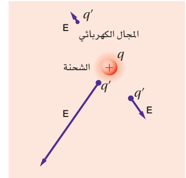
■ الشكل 1-6 تُستخدم الأسهم لتمثيل مقدار المجال الكهربائي المتولد حول شحنة كهربائية عند مواقع مختلفة، واتجاهه.
