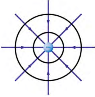
■ الشكل 6-7 فرق الجهد الكهربائي بين أي نقطتين على أي مسار دائري حول شحنة يساوي صفر.
