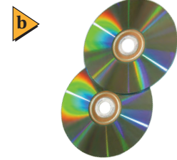
■ الشكل 12-4 جوهرة مصنوعة في صورة محزوز نفاذ تنتج أطيفاً ضوئية (a). تُعدّ الأقراص المدمجة محزوزات انعكاس؛ إذ تكوّن نمط طيف الحيود عندما يسقط عليها ضوء أبيض (b).
