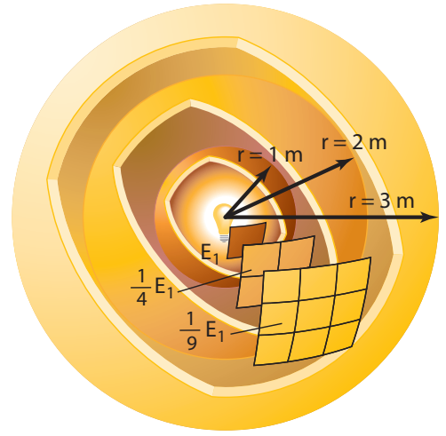
■ الشكل 5-1 تتغير الاستضاءة E الناتجة عن مصدر ضوء نقطي عكسيًا مع مربع البعد عنه.
