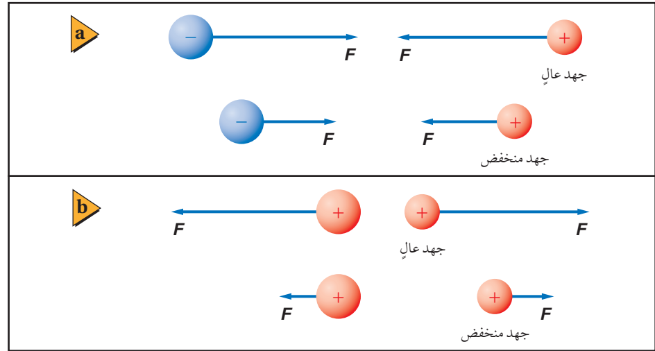
■ الشكل 6-8 في أثناء تقريب شحنة اختبار إلى شحنة مخالفة لها في النوع يقل الجهد عند مواقع شحنة الاختبار (a)، في حين يزداد الجهد عند مواقع شحنة الاختبار في أثناء تقريبها إلى شحنة مماثلة لها في النوع (b).
